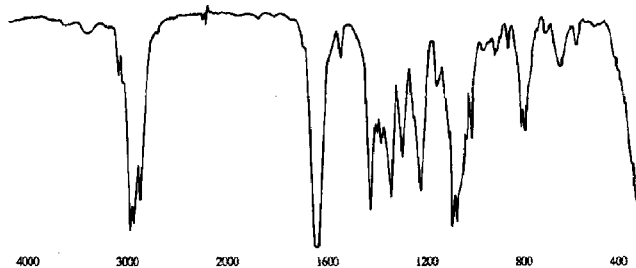
图 1 丁草胺的红外光谱图
